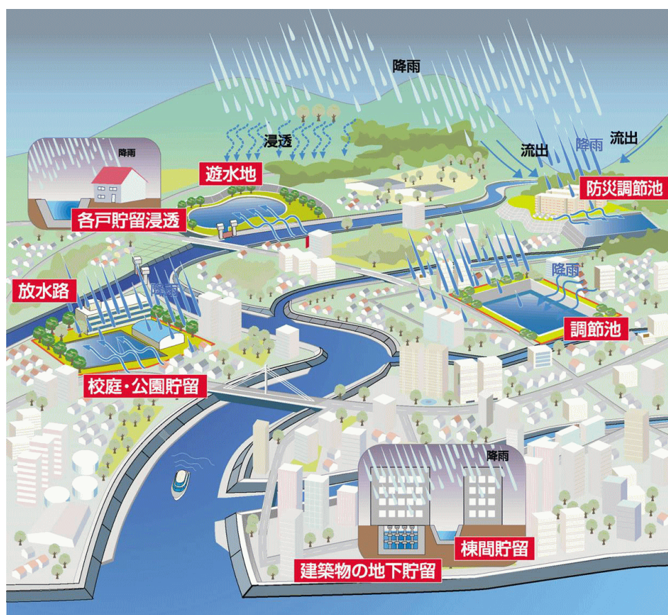
図 2 流域治水のイメージ図（国交省パンフ）より）
